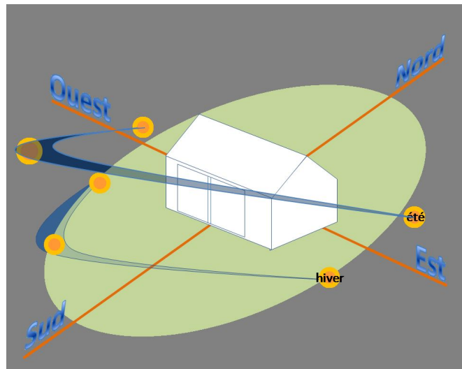
Implantation d'une construction par rapport à la course du soleil
