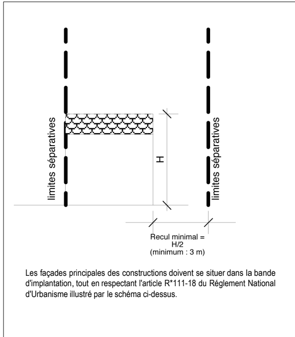
Implantation d'une construction sur sa parcelle
